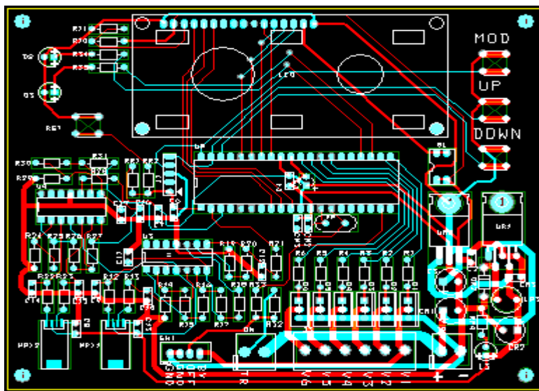
Hình 3.13 Sơ đồ mạch in mạch theo dõi áp lực, điều khiển hệ thống
