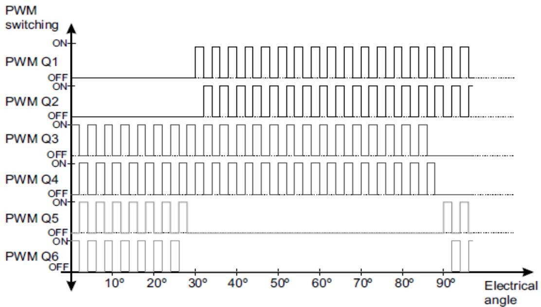
Hình 3.4 Giản đồ xung đóng ngắt tăng công suất kiểu độc lập
